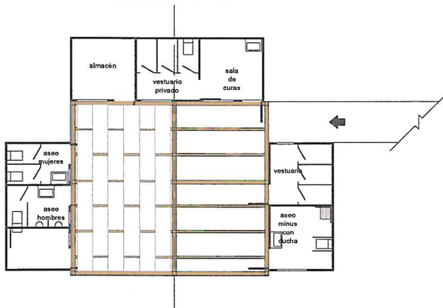
Punto Iglesia PLANTA DE TECHO
