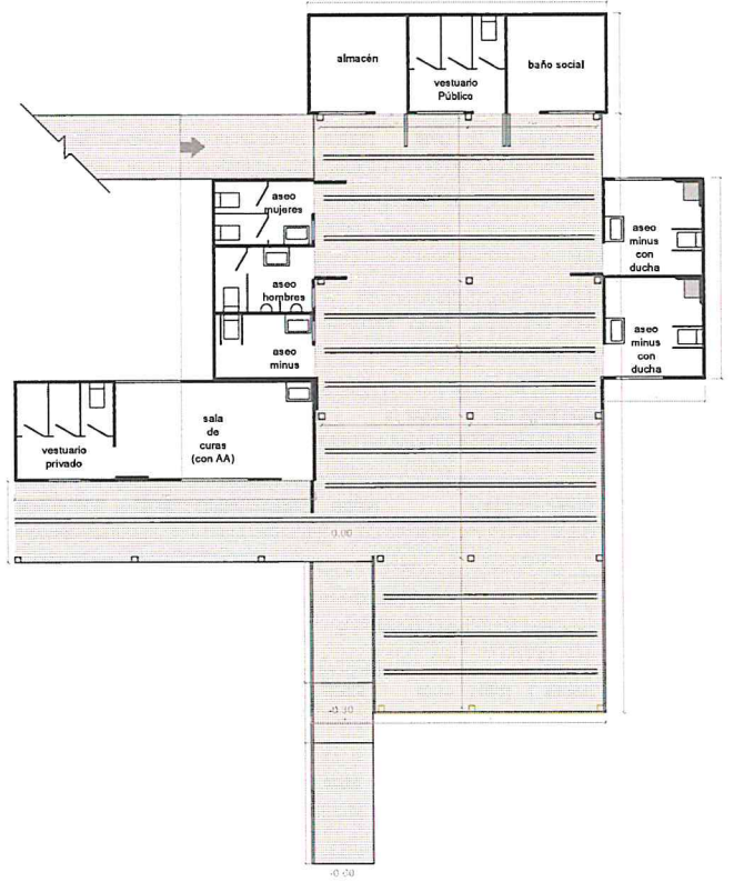
Punto Maraute PLANTA DE SUELO
