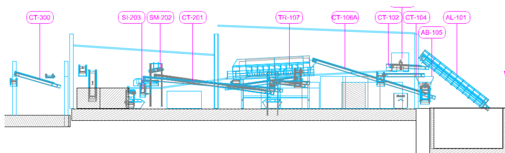
Figura 11. Nave metálica. Proyecto original.
