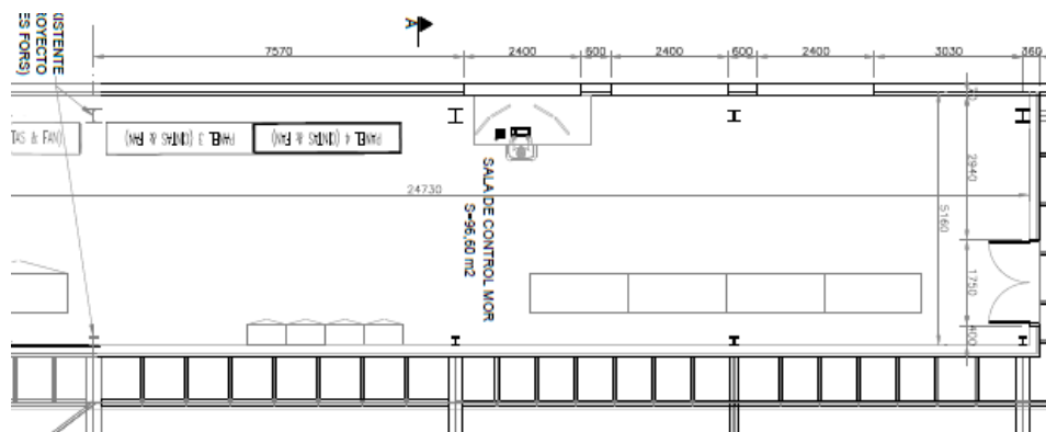
Figura 14. Sala control. Proyecto final.
