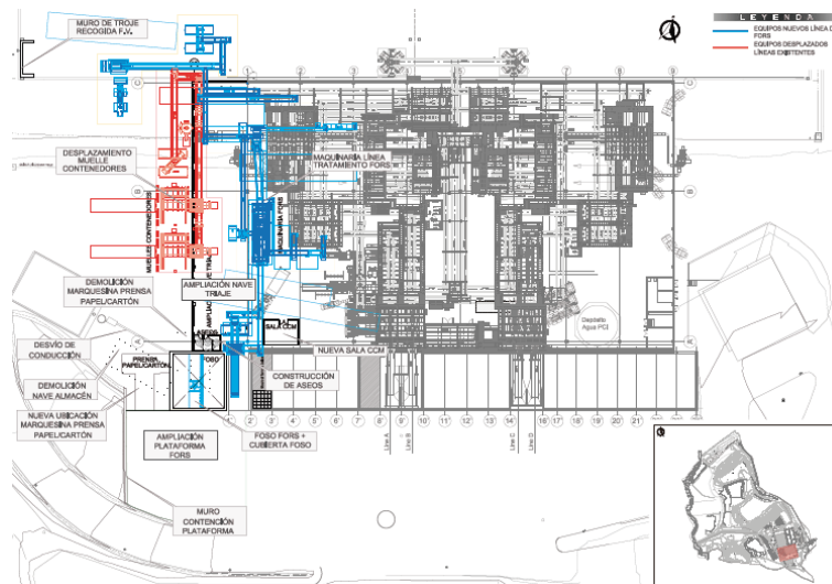
Figura 2. Distribución inicial del proyecto (en color azul).
