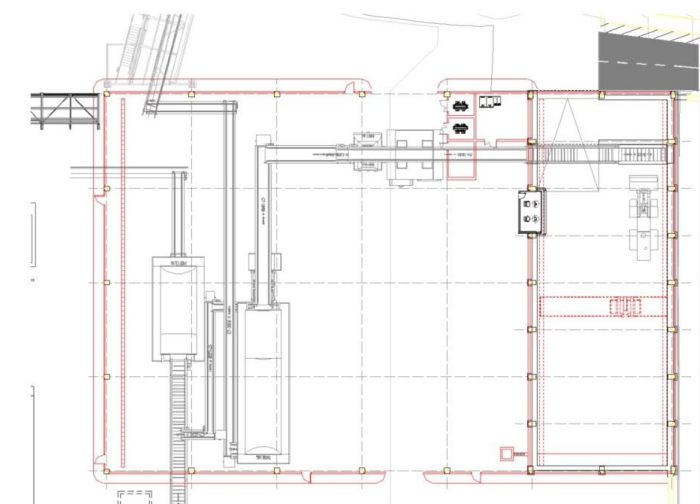
Figura 3. Distribución final del proyecto.
