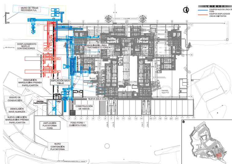
Figura 9. Distribución inicial del proyecto.
