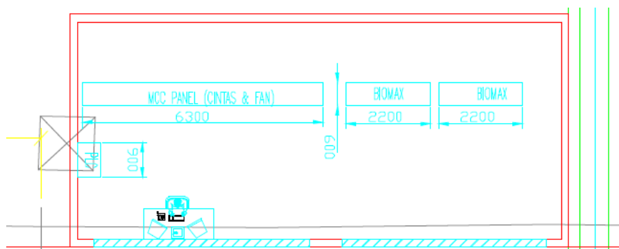
Figura 6. Sala control. Proyecto original.
