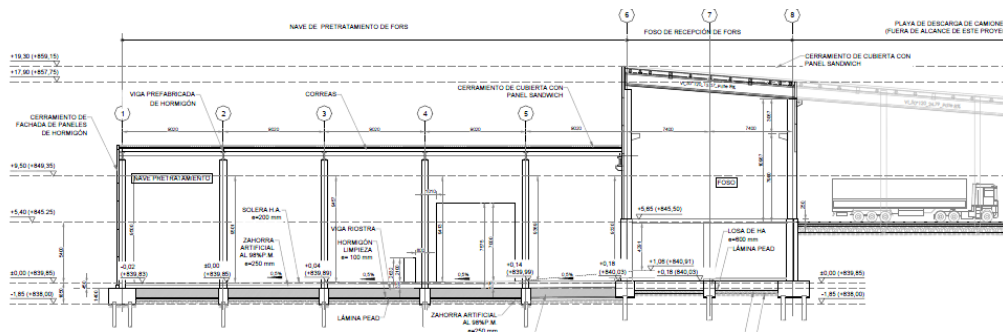
Figura 12. Nave hormigón prefabricado. Proyecto final.
