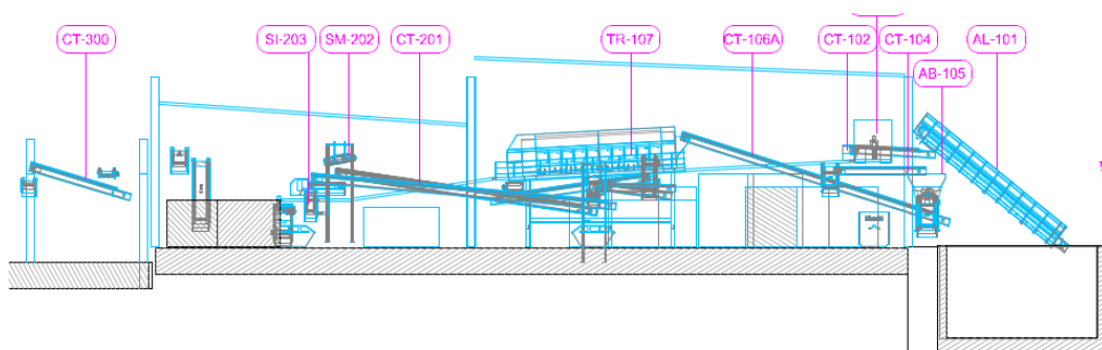
Figura 4. Sección Ampliación de nave. Proyecto original.
