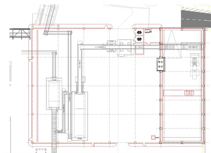
Figura 10. Distribución final del proyecto.
