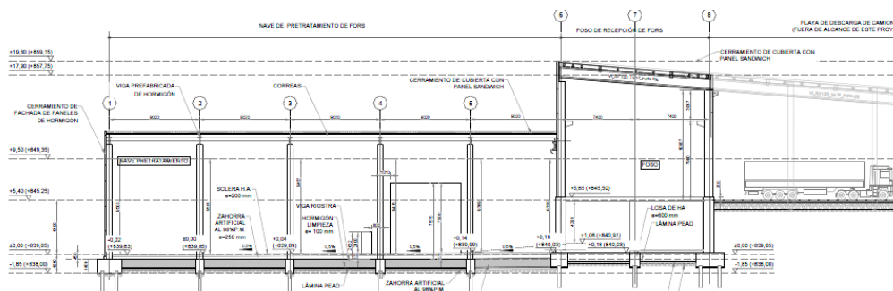
Figura 5. Nave hormigón prefabricado. Proyecto final.
