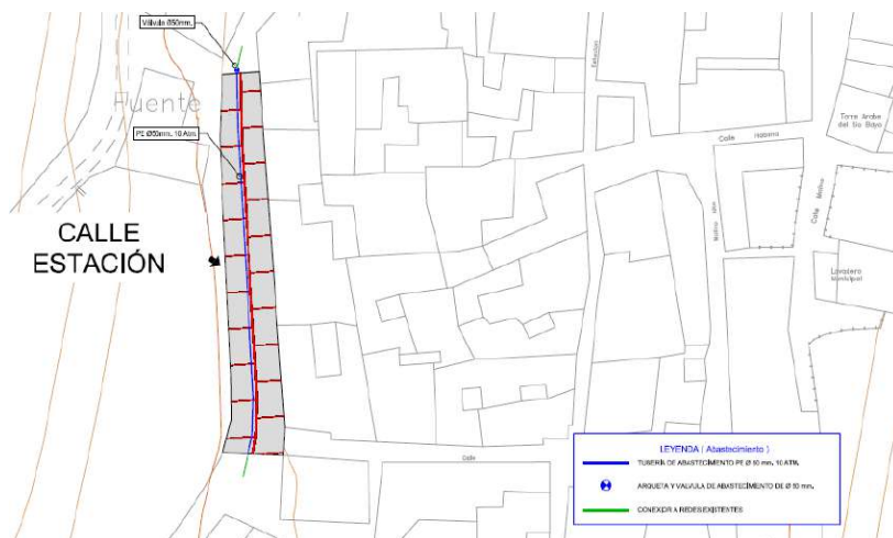
Planta proyectada Calle Estación
