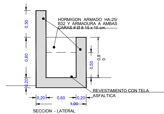
DEFINICION GEOMETRICA
