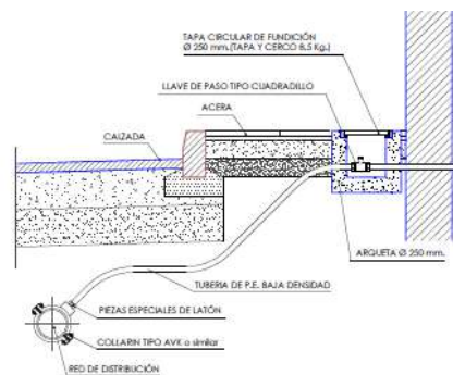
Detalle de acometidas domiciliarias de abastecimiento
