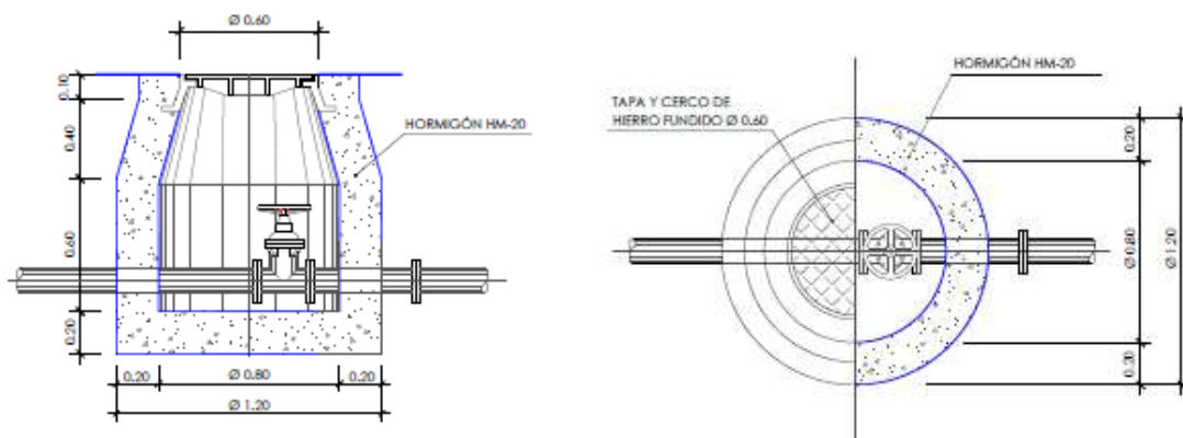
Detalle de las válvulas a colocar
