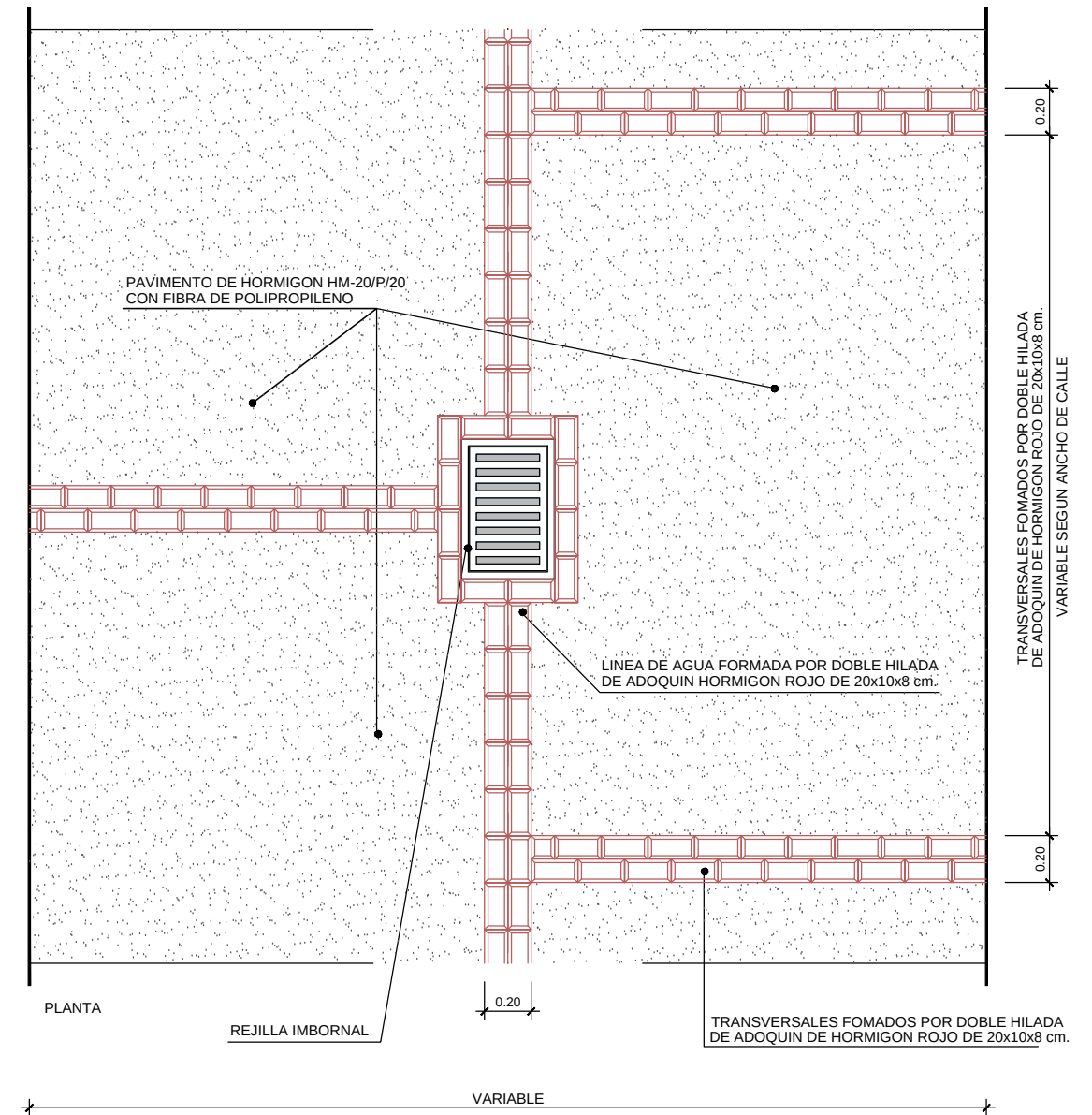
PLANTA-SECCIÓN
