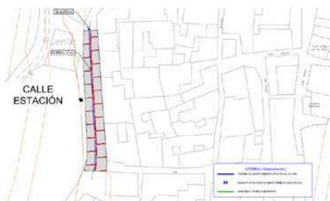
Planta proyectada Calle Estación
