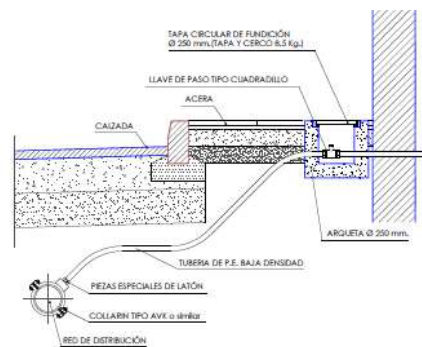
Detalle de acometidas domiciliarias de abastecimiento
